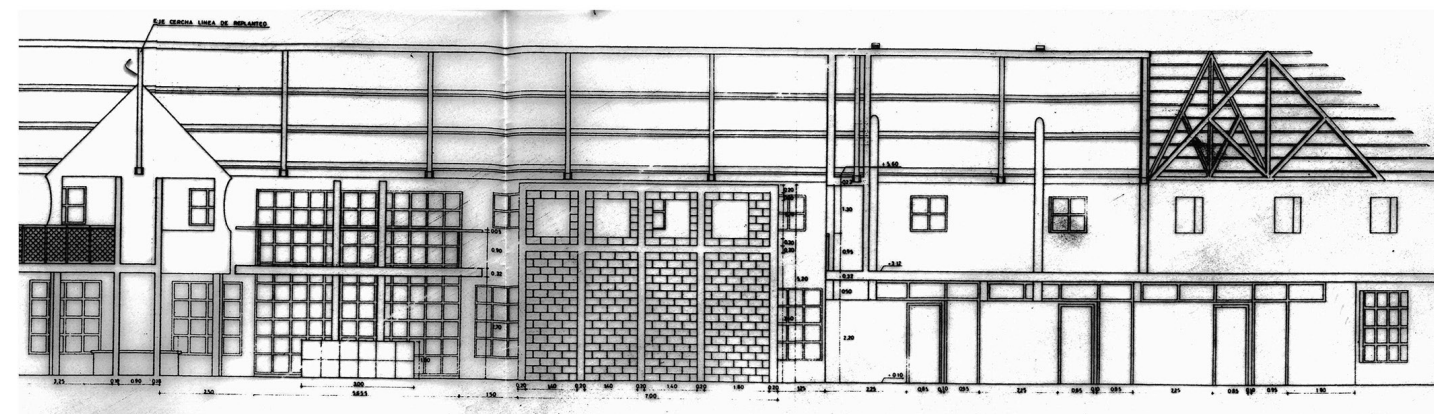
Sección transversal de la Biblioteca Municipal (1982).
