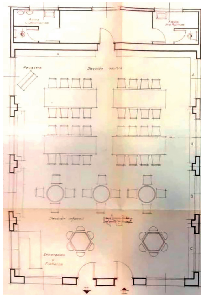
Plano de planta de la Biblioteca Municipal habilitada en el Lavadero Público (1963).
